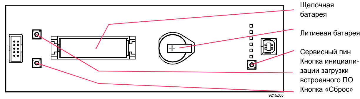
PXC36....D, PXC36-E.D
